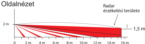
Oldalnézet
